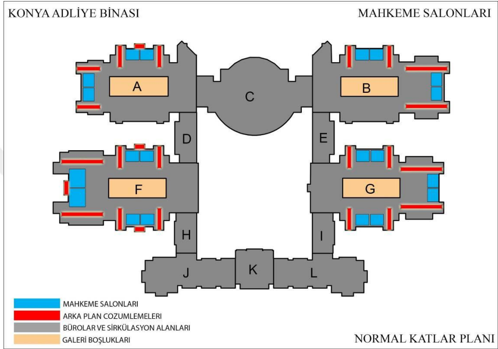
Şekil 5.50. Konya Adliye Binası Arka Plan Çözümlerleri
