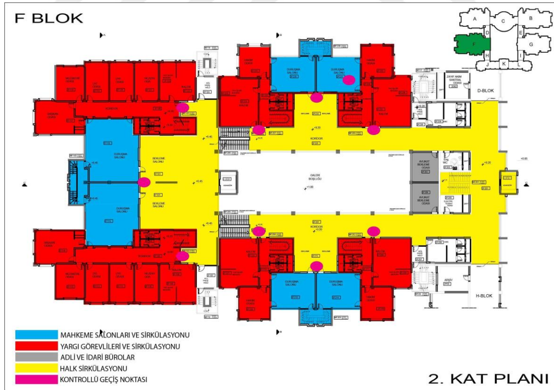
Şekil 5.38. F Blok Normal Katlar Ön Plan- Arka Plan Analizi
