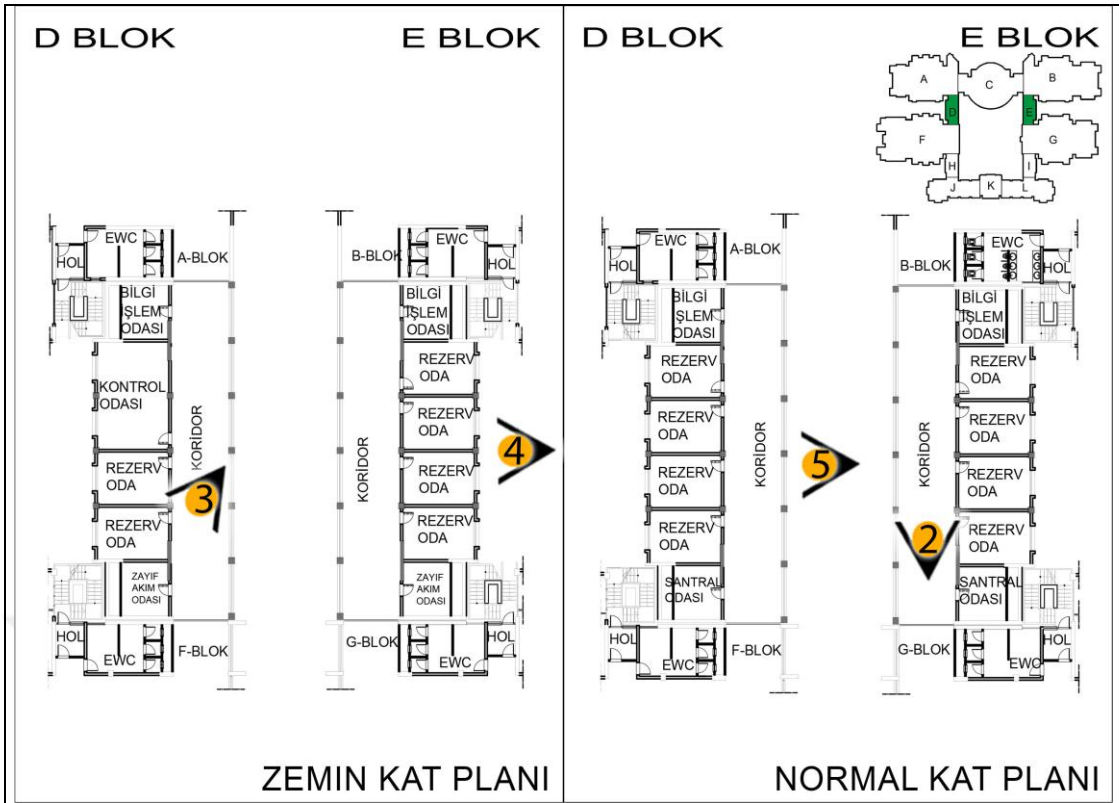
a- Kat planları
