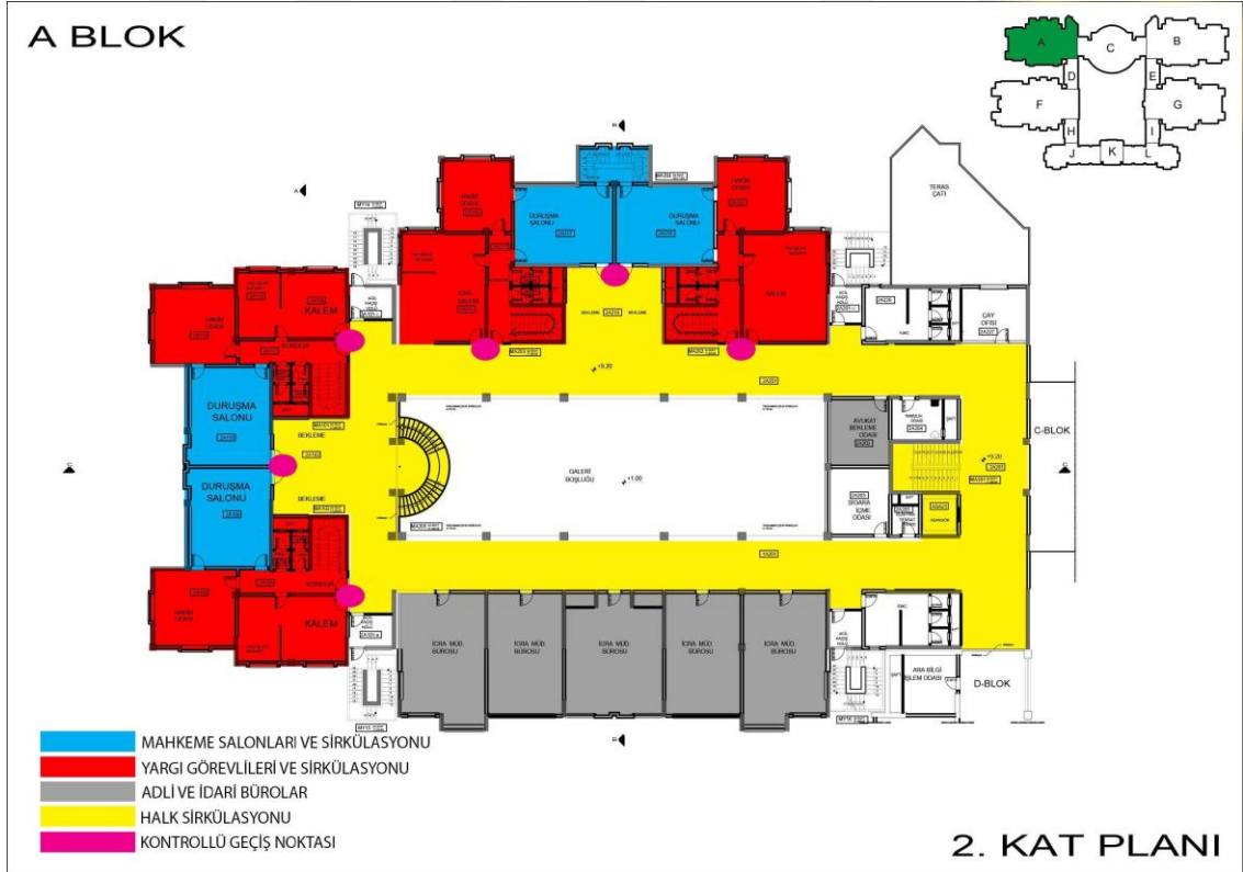
Şekil 5.20. A Blok Normal Kat Ön Plan- Arka Plan Analizi
