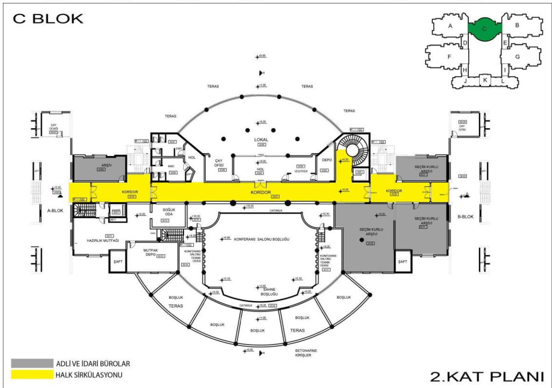
Şekil 5.31. C Blok Normal Kat Ön Plan- Arka Plan Analizi
