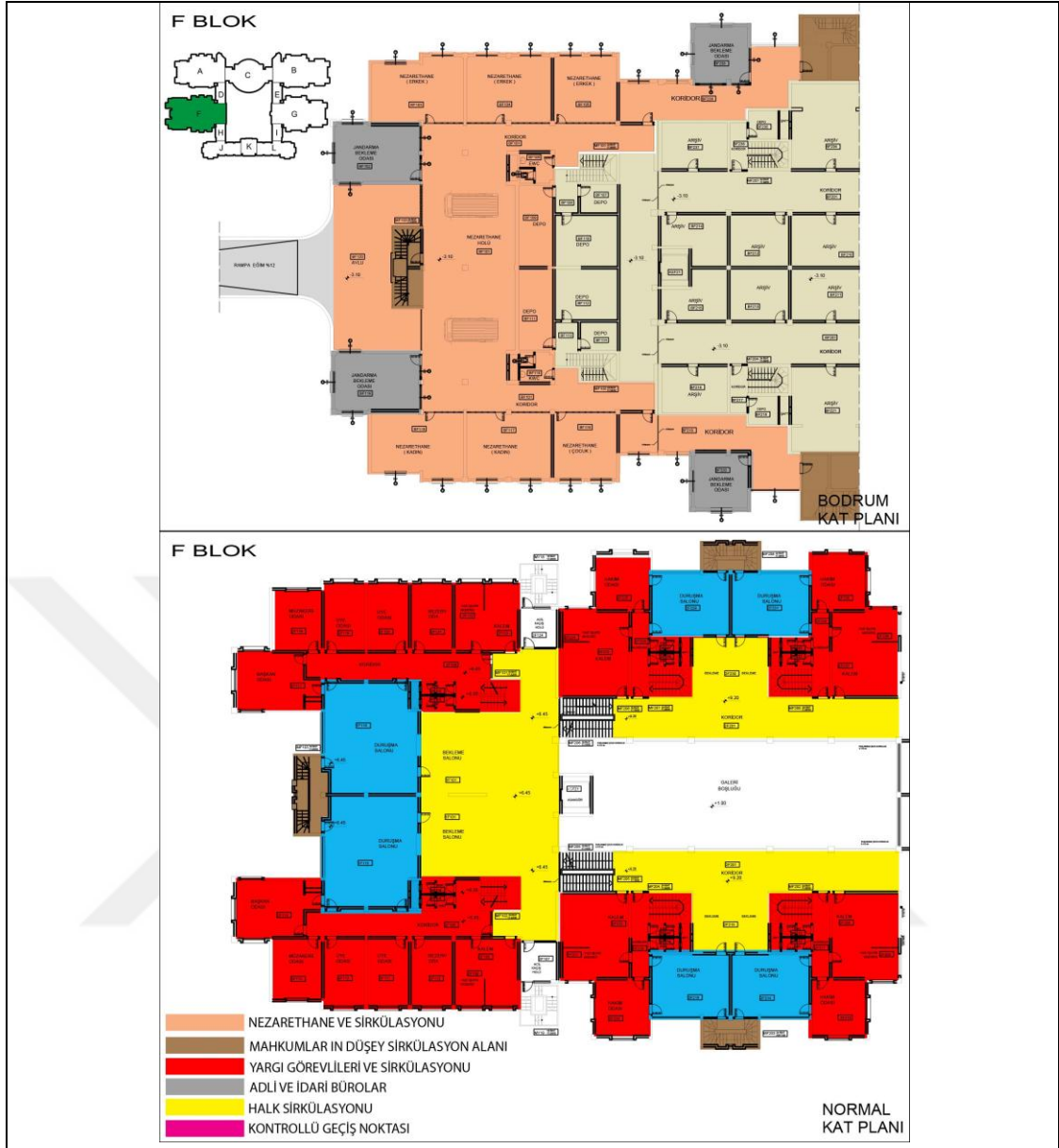
a- F Blok Nezarethane Planı
