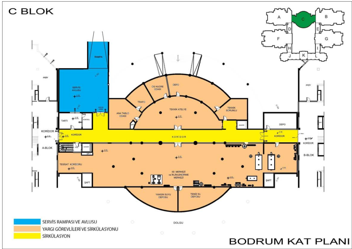
Şekil 5.27. C Blok Bodrum Kat Planı
