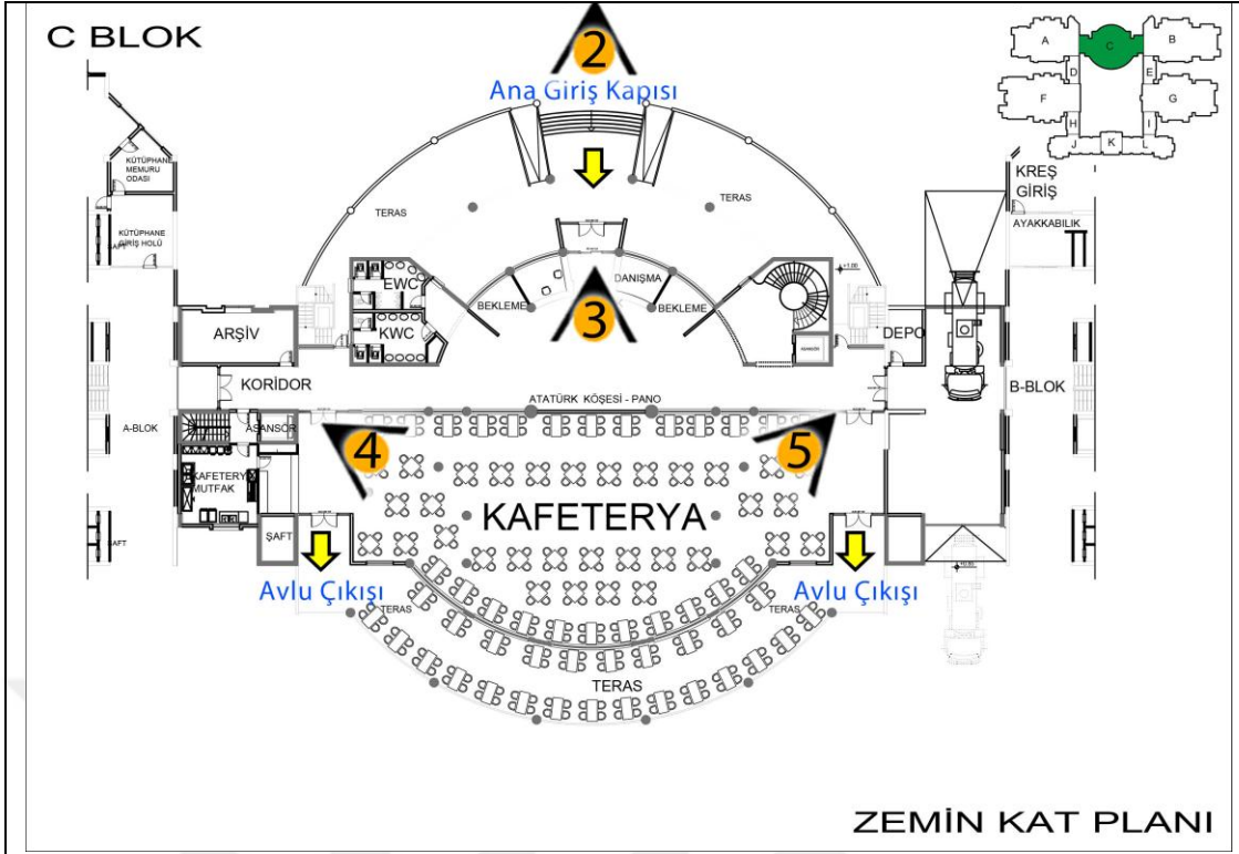
a- Zemin Kat Planı
