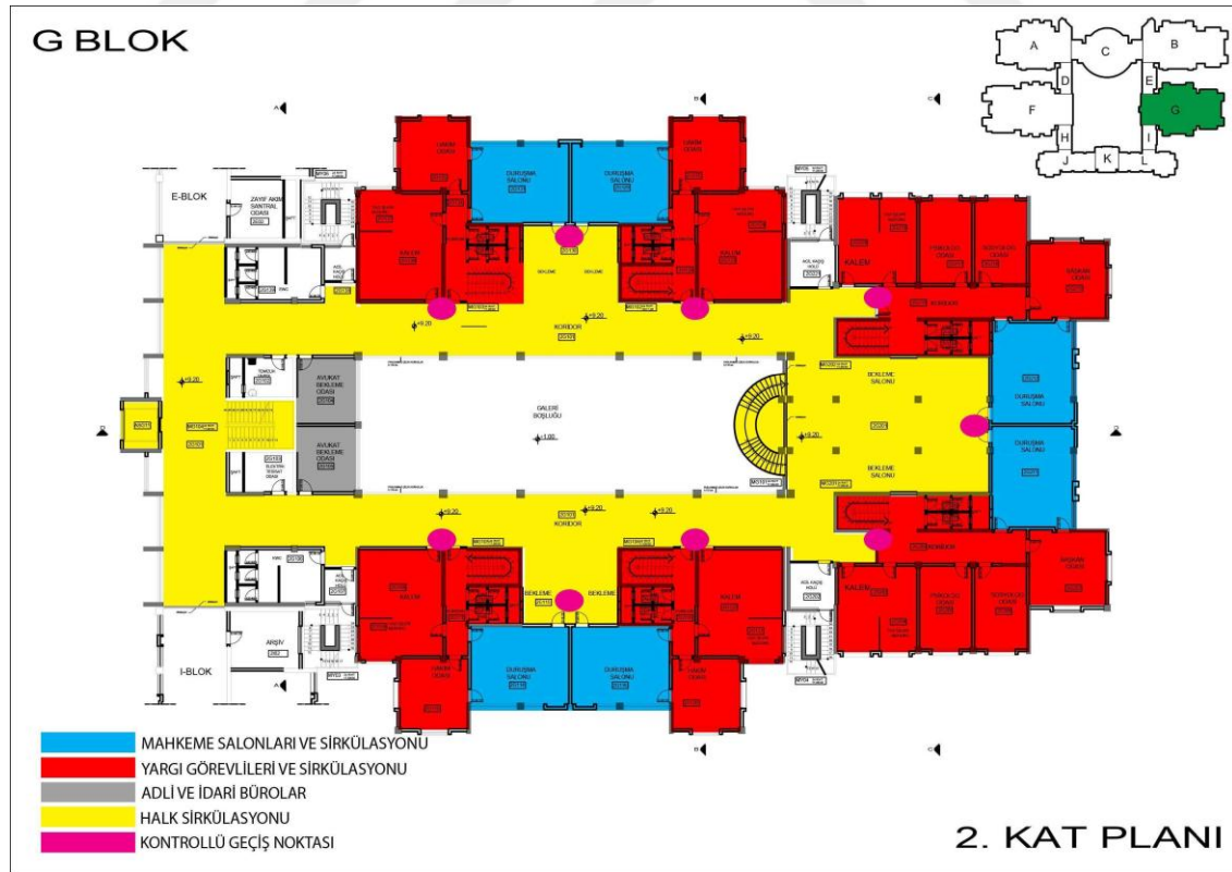
Şekil 5.43. G Blok Normal Katlar Ön Plan- Arka Plan Analizi
