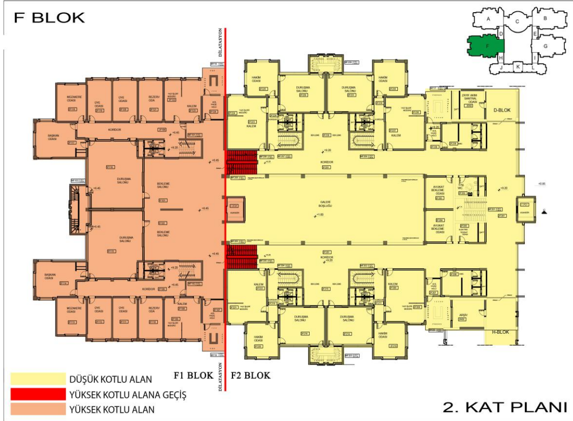
Şekil 5.36. F Blok Kot Farkı Planı
