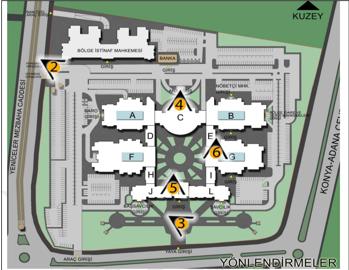
a- Yönlendirmeler Planı
